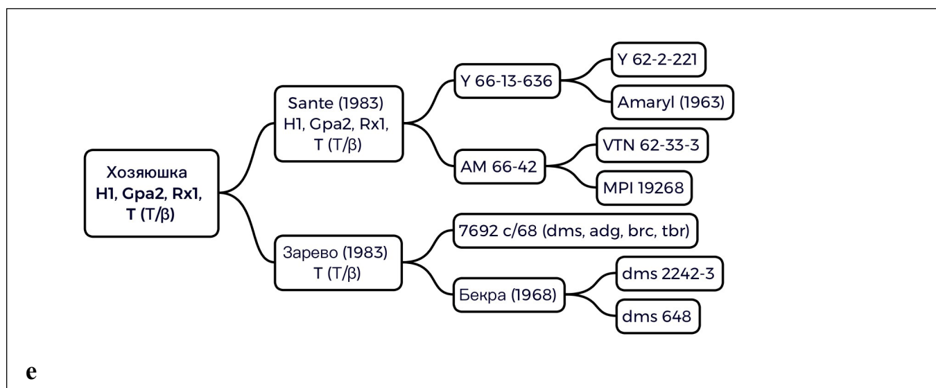
Рис. 2. Родословные сортов селекции Омского АНЦ. (a) ‘Алена’, (b) ‘Былина Сибири’, (c) ‘Вечерний Омск’, (d) ‘Триумф’, (e) ‘Хозяюшка’
